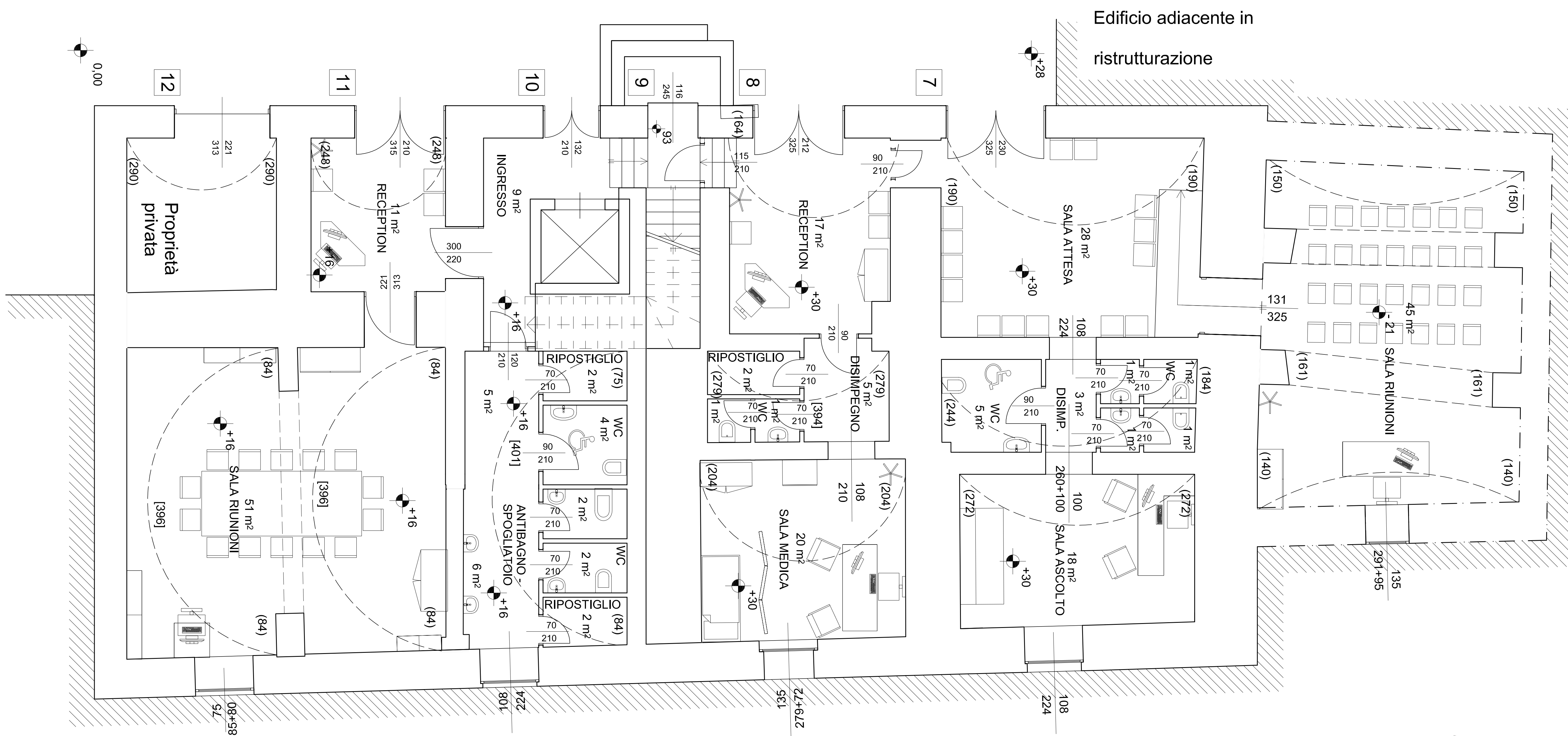
PIANO TERRA CENTRO ANTIVIOLENZA (con quote) Rapp. 1:50
